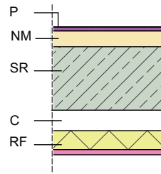
Figura 3.4.1 Falso techo
