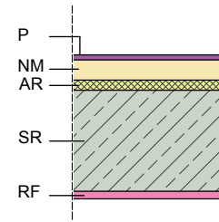
Figura 3.4.2 Aislante a ruido de impacto
