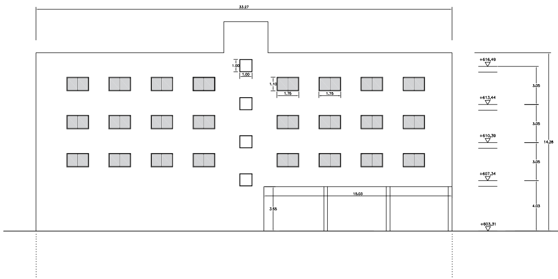
Figura 5.7 Alzado norte
