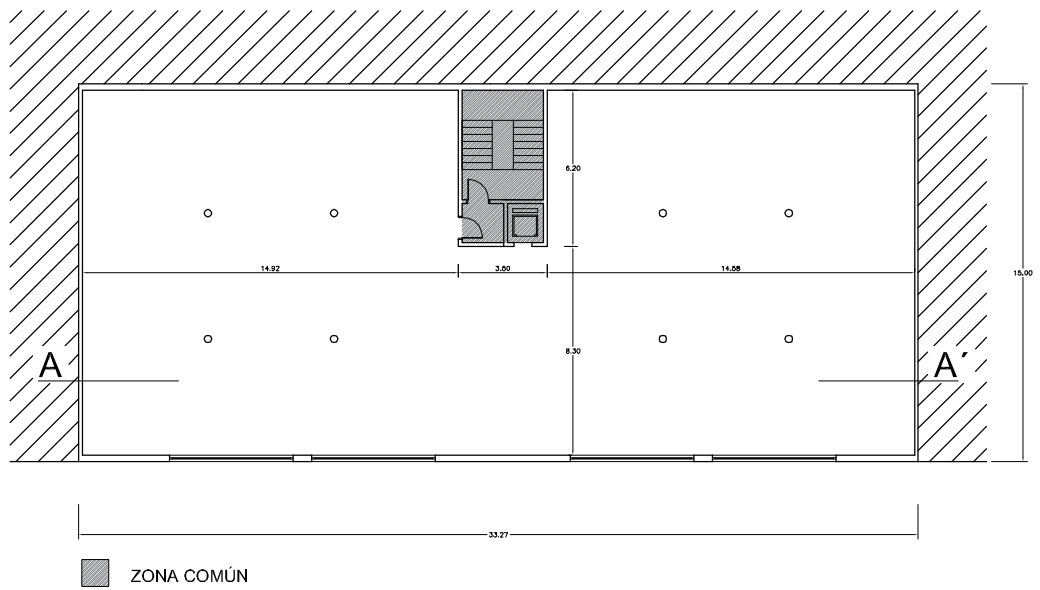
Figura 5.1 Planta sótano
