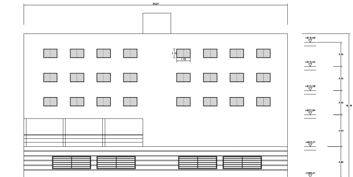
Figura 5.6 Alzado sur
