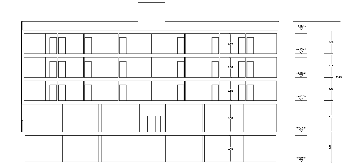
Figura 5.4 Sección A-A'
