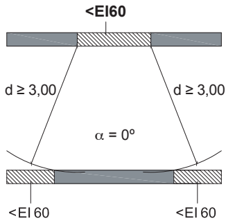
DB SI 2 Figura 1.1 Fachadas enfrentadas
