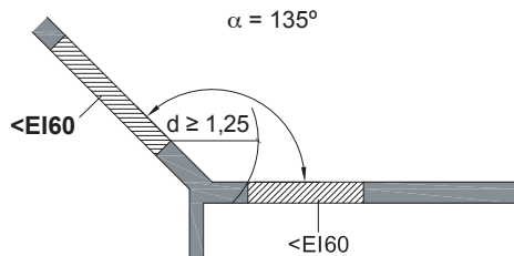
DB SI 2 Figura 1.5 Fachadas a 135°
