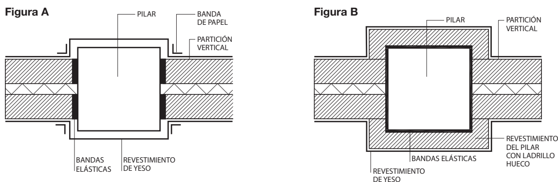
Figura 4.6. Ejemplo encuentro partición vertical de dos hojas con pilar
