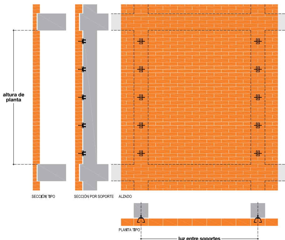
Figura A.1. Esquema de cerramiento sustentado en forjados y soportes
