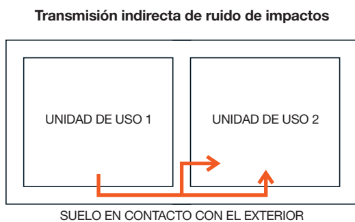
Figura 3.8.3 Transmisión de ruido de impactos entre recintos colindantes horizontalmente
