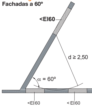
DB SI 2 Figura 1.3 Fachadas a 60°
