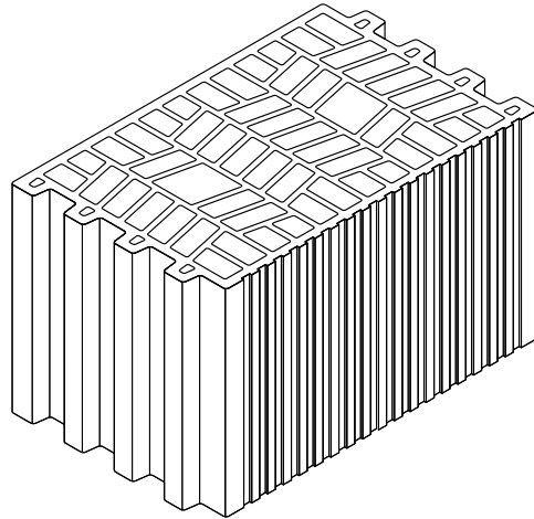
Figura 2.7 Bloques cerámico aligerado machihembrado
