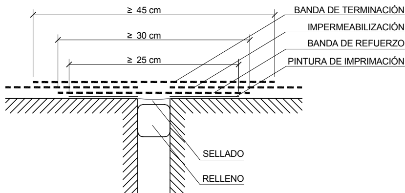
DB HS 1 Figura 2.2 Ejemplo de junta estructural
