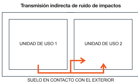
Figura 3.7.2 Transmisión de ruido de impactos entre recintos colindantes horizontalmente
