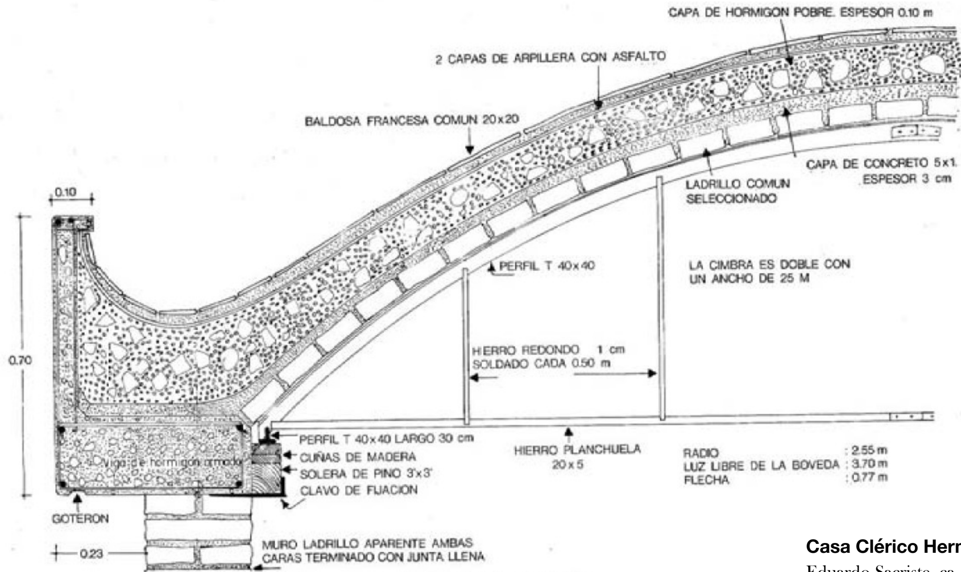
Fig. 84. Detalle de bóveda y cimbra.
